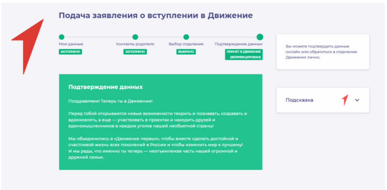
Рисунок 3 – Подтверждение данных.
