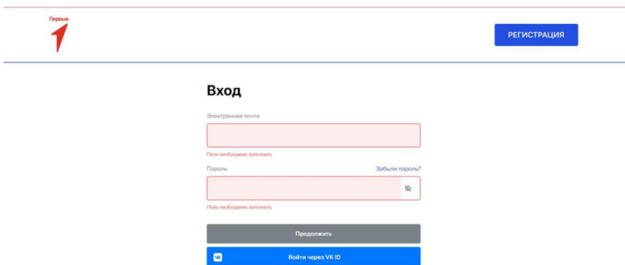
Рисунок 3 – Авторизация
