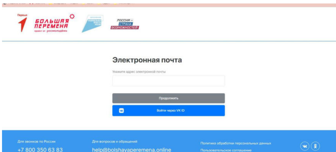
Рисунок 2.1 - Регистрация
